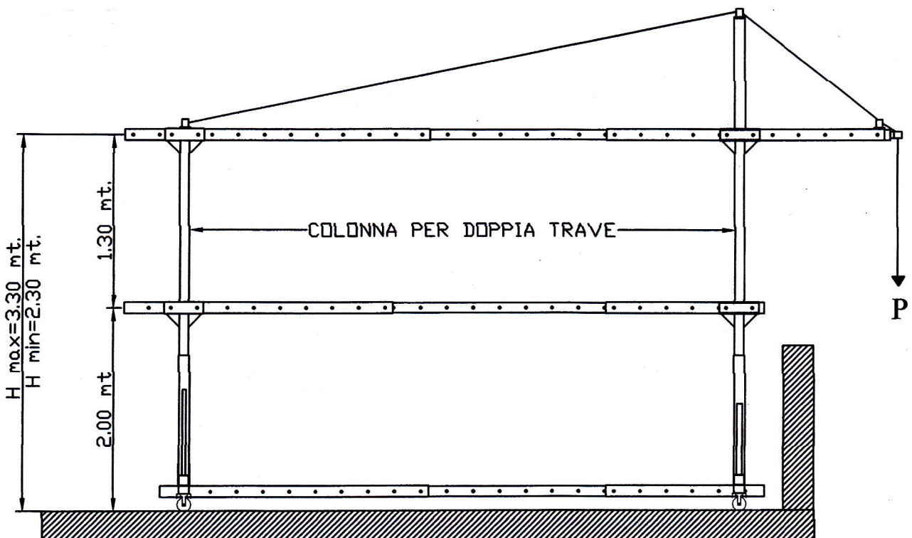
SCHEMA DOPPIA TRAVE
