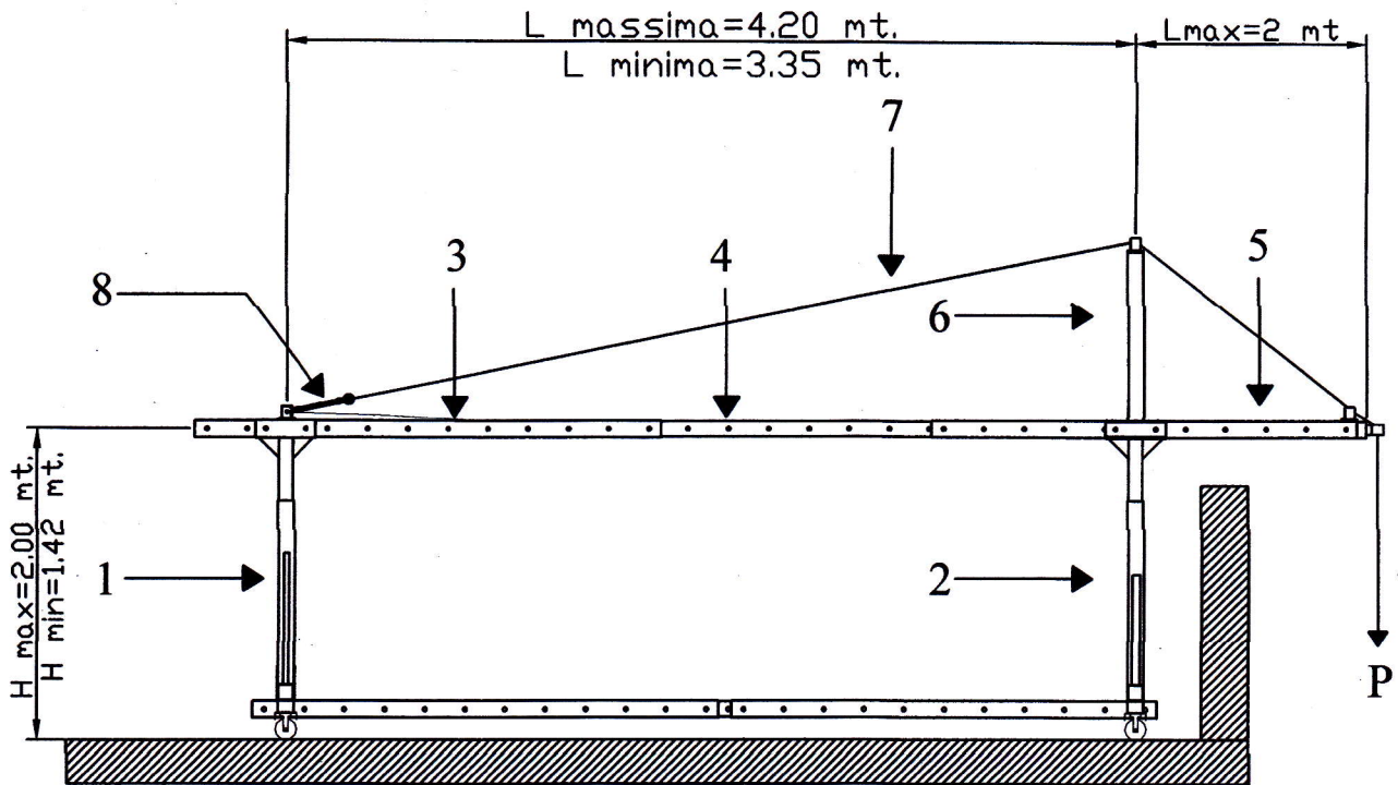
SCHEMA SOSPENSIONE SEMPLICE
